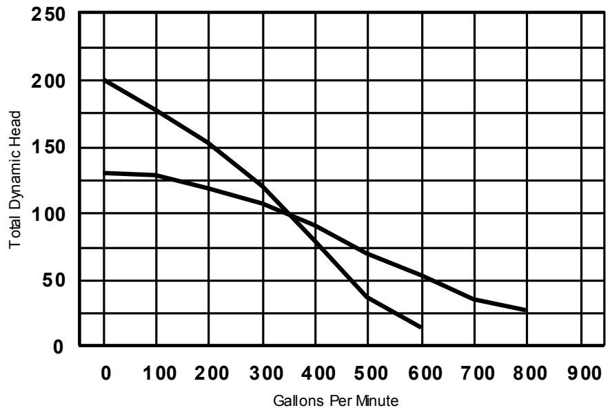
Piranha Model PP-1500 HV & HH 15 HP - 230/460 Volt
